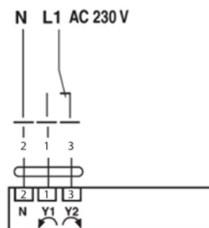
Управление двухпозиционным регулятором
