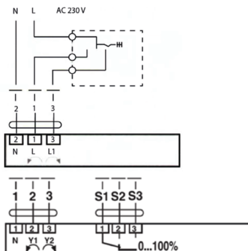
Трёхпозиционное устройство управления
